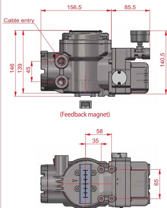
ASD-7001 Linear type
